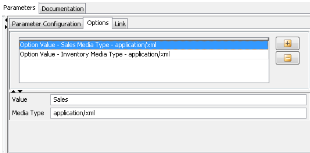
Figure 15: Parameter Configuration
